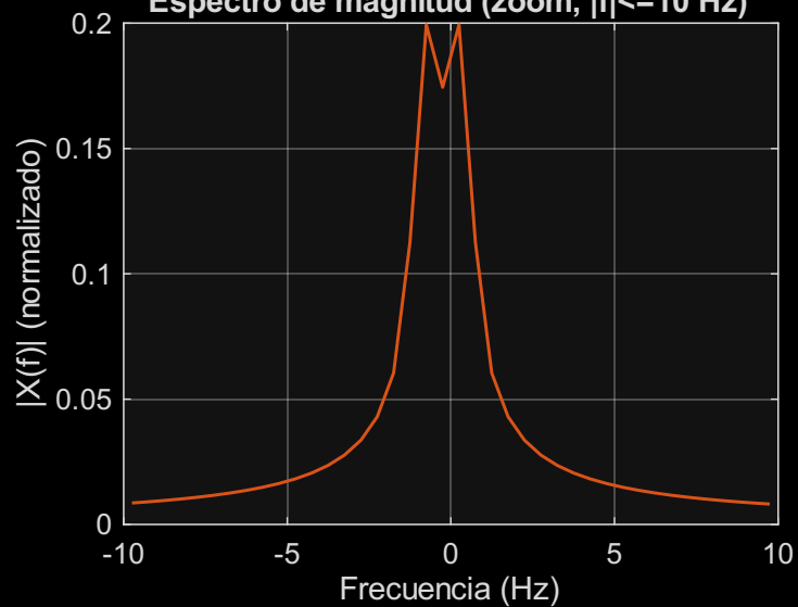
Espectro de magnitud (zoom, |f| \leq 10 Hz)
